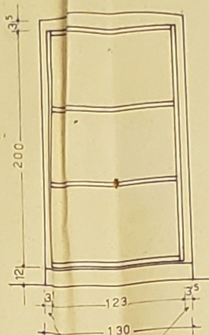
CONFEÇÃO DO CHASSIS DO PAINEL (MEDIDAS A SEREM ADOPTADAS).
