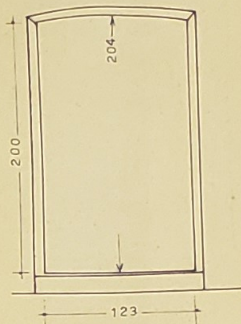
CONFEÇÃO DA FOLHA DE COMPENSADO (MEDIDAS A SEREM ADOPTADAS).
